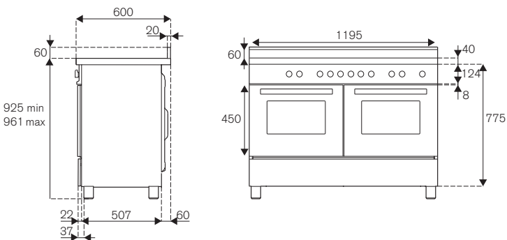
PRO126G2EART
