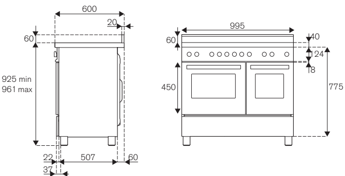
PRO105I2EGIT PRO105I2EART
