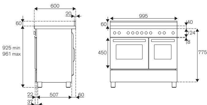
PRO106L2EART
