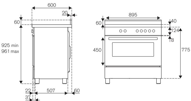
PRO95I1EGIT PRO95I1EART
