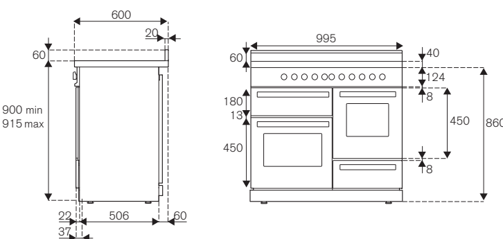
PRO106L3EART
