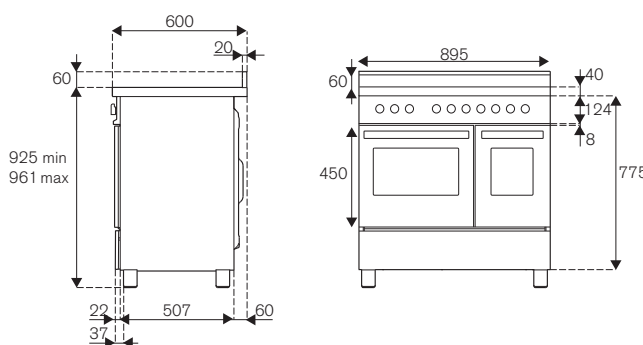
PRO96L2EART
