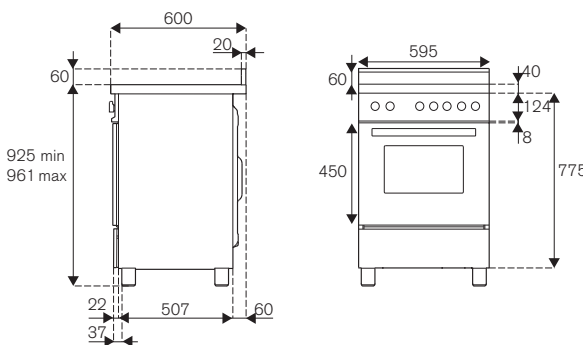
PRO64I1EGIT PRO64I1EART
