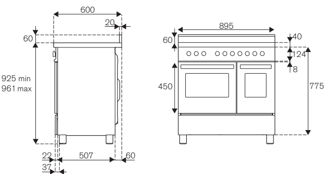
PRO95I2EGIT PRO95I2EART
